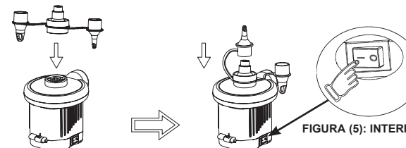
FIGURA (6): CONECTE LA BOQUILLA
